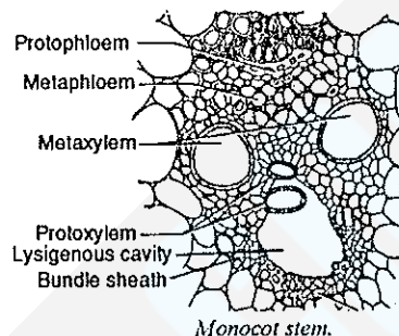
Monocot stem.
